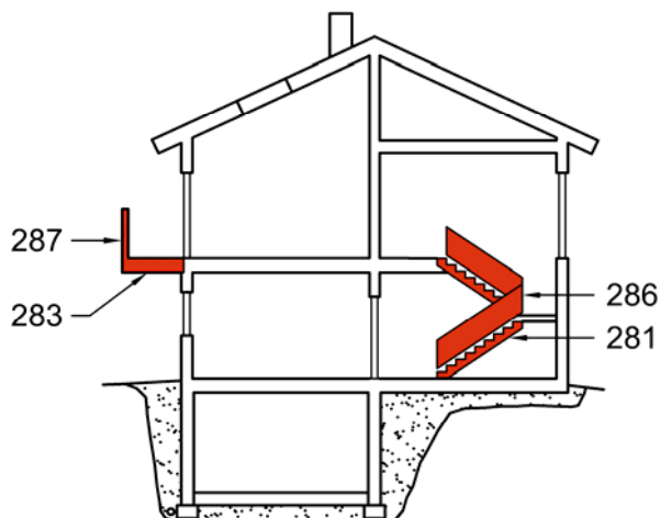
Figur 6 Bygningsdel 28: Trapper, balkonger m.m.
